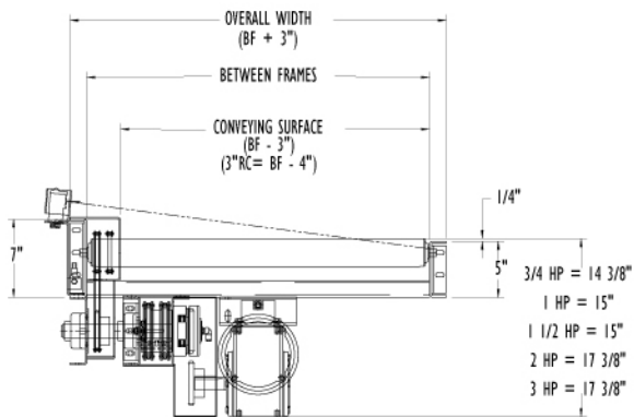
SZA25 ICDA AIR CLUTCH UNDERNEATH
